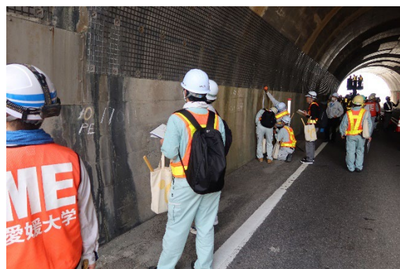
トンネル（砥鹿山隧道）
