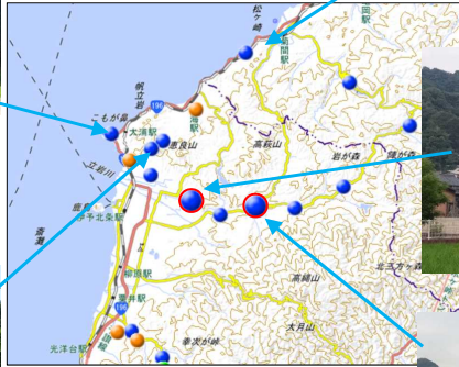
みかん畑・道路斜面の崩壊(下難波地区)
