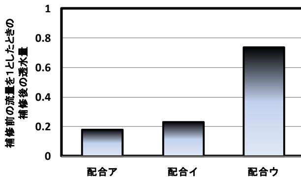
図-9 透水試験結果
